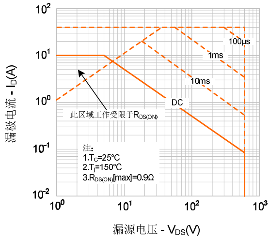
图9-1. 最大安全工作区域 (SR 10N65F)
