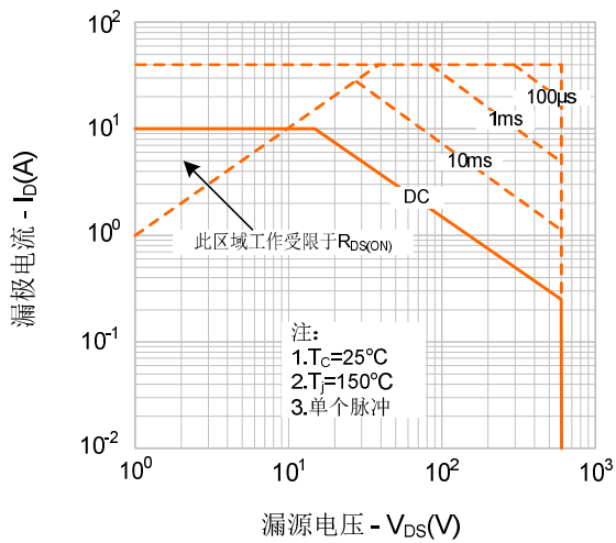
图9-3. 最大安全工作区域 (SR 10N65S)
