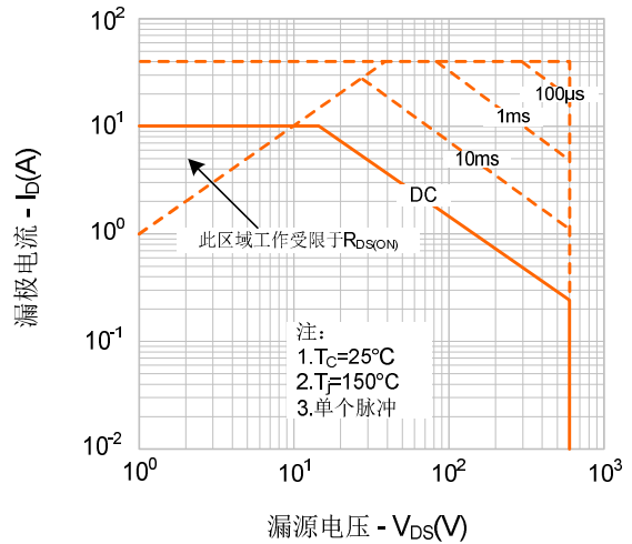
图9-2. 最大安全工作区域 (SR 10N65T/D)
