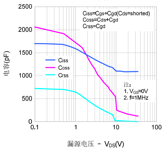
图5. 电容特性
