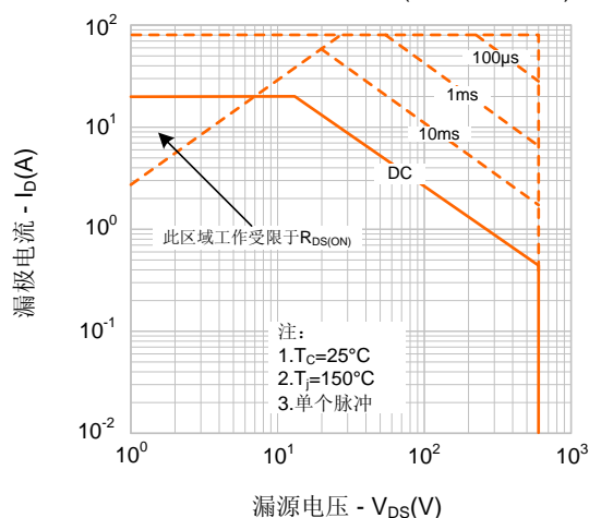
图9-2. 最大安全工作区域( SR20N60P )
