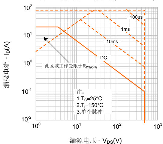
图9-1. 最大安全工作区域( SR20N60T)
