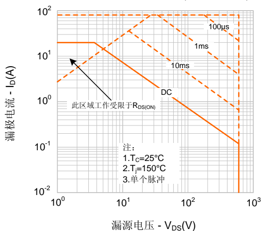
图9-1. 最大安全工作区域( SR20N60F)
