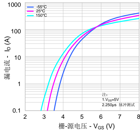
图 2. 传输特性
