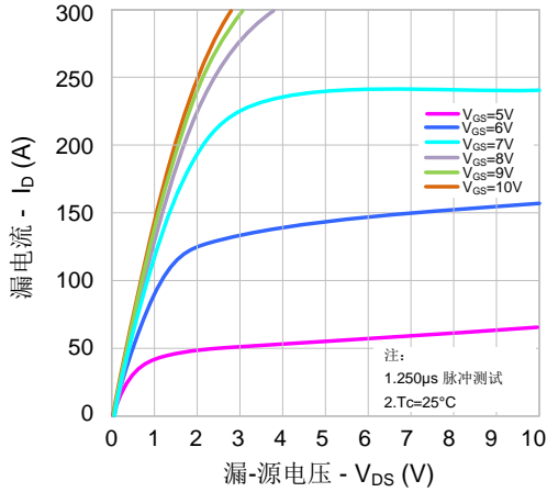
图 1. 输出特性
