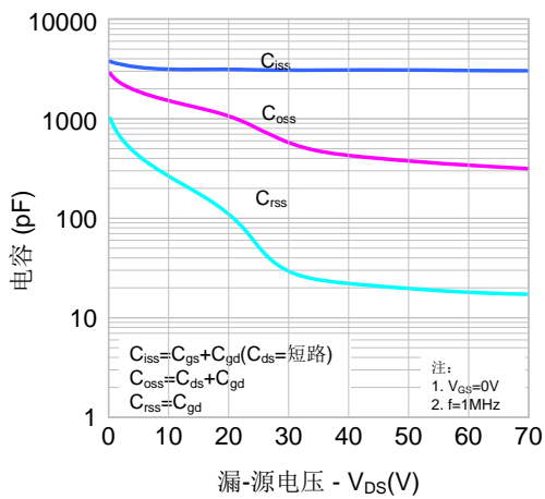
图 5. 电容特性
